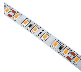
KANLUX Pásek LED SMD teplá bílá 16W/m 270lm/m 24V 3000K IP00 5m ELFETEX kód: 11.419.649 Kód výrobce: 33311
